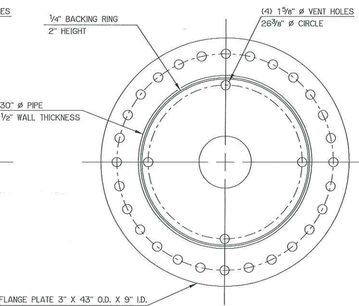
FLANGE PLATE 'B'
